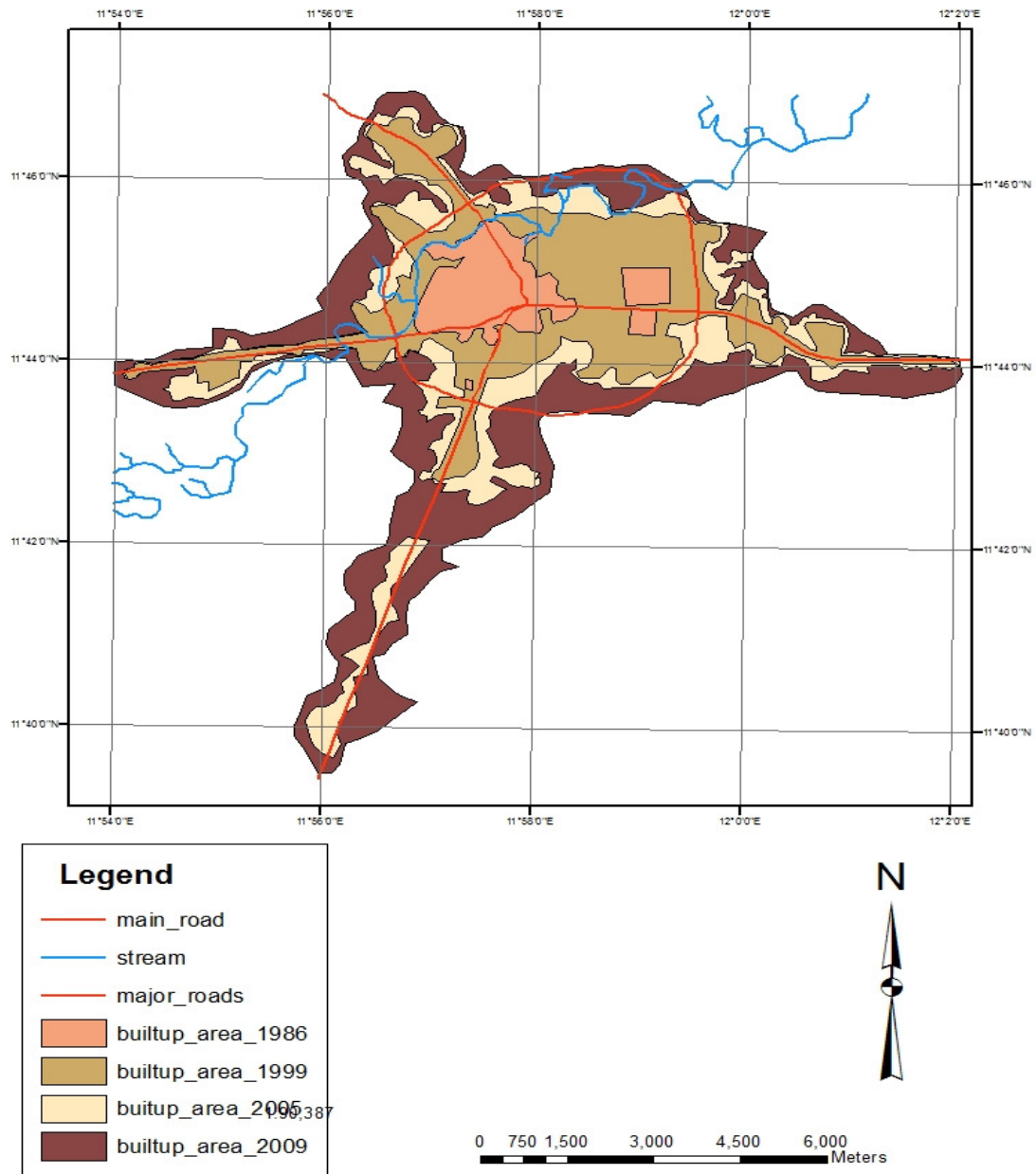
Fig. 5. Damaturu landuse/landcover changes
