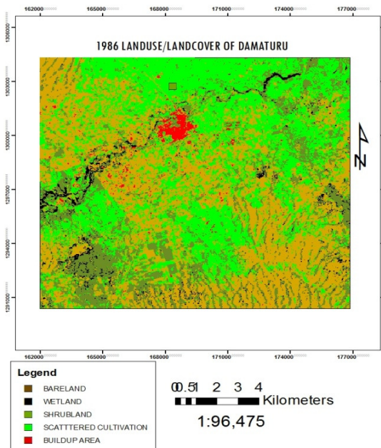
Fig. 3.1 1986 LULC of Damaturu
